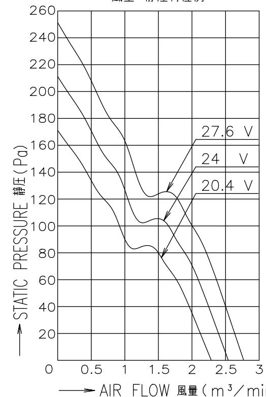
風量-静圧特性例
