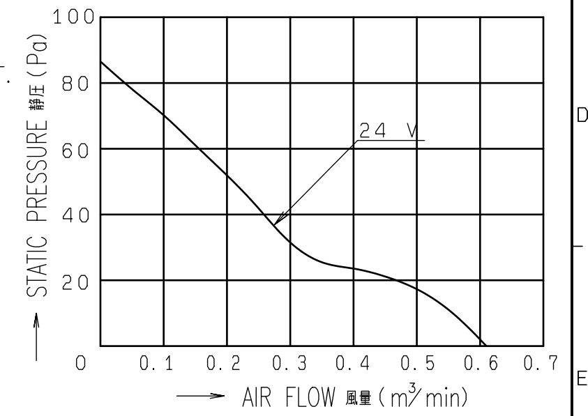
風量-静圧特性例
