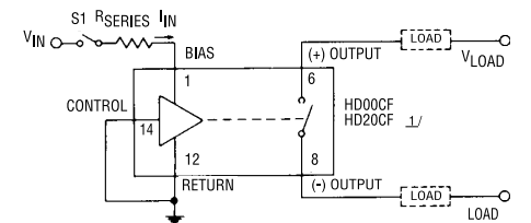
(D) 2 TERMINAL INPUT (DIRECT DRIVE)
