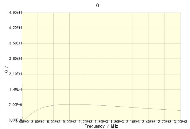
MLF2012C220KT000
