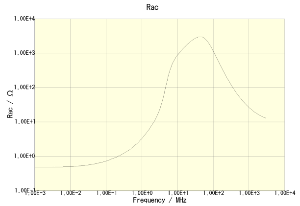
MLF2012C220KT000
