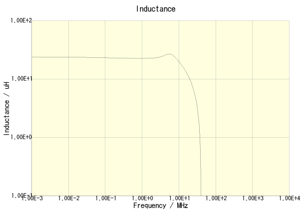
MLF2012C220KT000
