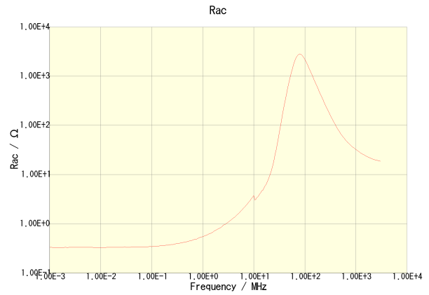
MLF2012A3R3KT000
