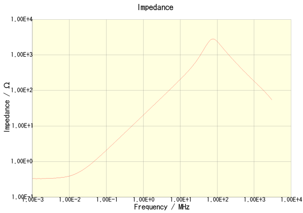
MLF2012A3R3KT000
