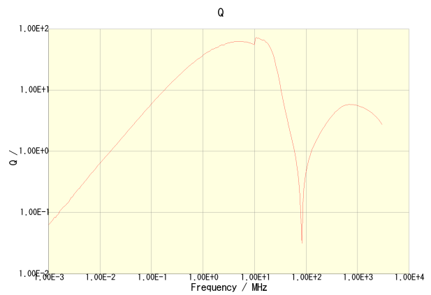
MLF2012A3R3KT000
