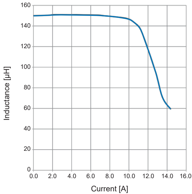
SPFC-EER28-125
