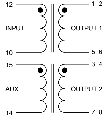
SLLC-ETD44
