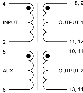
SLLC-ETD39
