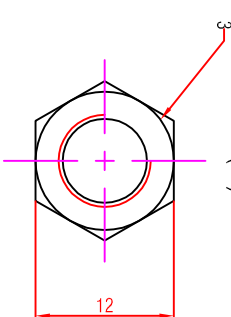
Nut (x2)
