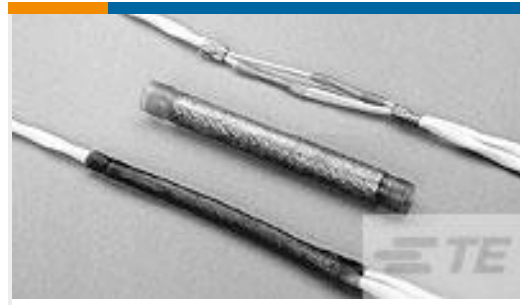
TE Part #621207-000 D-150-0174
