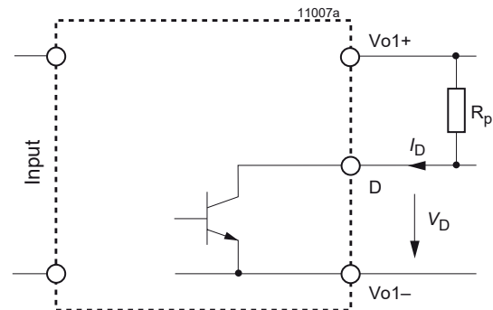
Fig. 21 Options D5 – D9, NPN output
