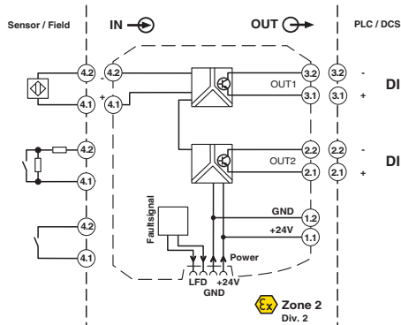
Blockschaltbild
