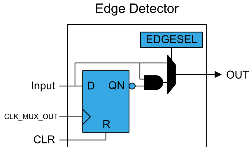
Figure 28-6. Edge Detector
