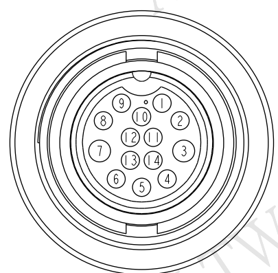
14 Brown/White 棕/白 13 Black/White 黑/白 12 Light Green 淺綠 11 Pink 粉紅 10 White 白 9 Gray 灰 8 Purple 紫 7 Blue 藍 6 Green 綠 5 Yellow 黃 4 Orange 橘 3 Red 紅 2 Brown 棕 1 Black 黑 Conn. Wire Color Pin Out
