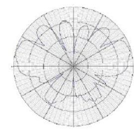
OD49M-6 E-Plane
