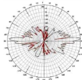
OD49M-11D1 E-Plane
