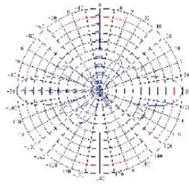
OD24M-7 E-Plane
