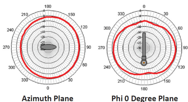
880 MHz
