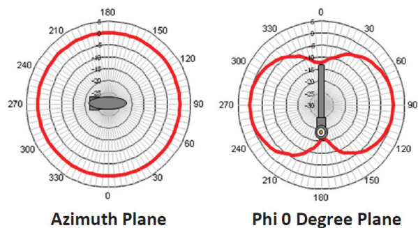
698 MHz
