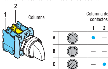
Accionamiento contactos en selector de 3 posiciones
