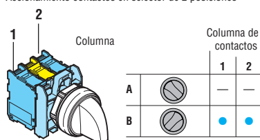
Accionamiento contactos en selector de 2 posiciones
