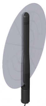
YZ-Plane Gain
