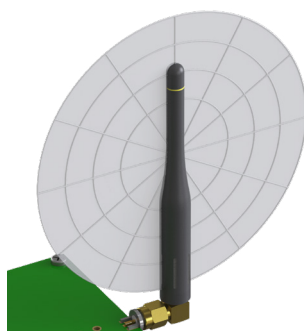
YZ-Plane Gain
