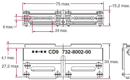
732-8002-00 4 Module Version
