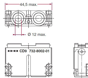
732-8002-01 2 Module Version
