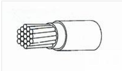
TE Part #732994-001 22759/43-16-9
