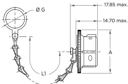
TYPE 76 -**
