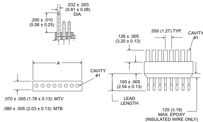
Receptacle
