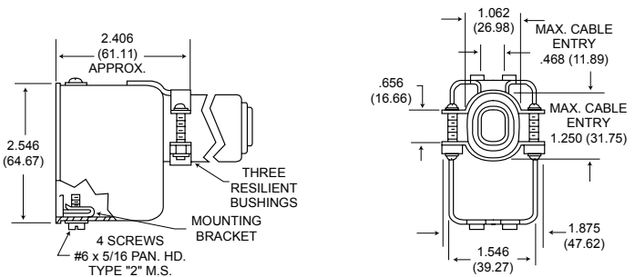
DPD2 19941-2
