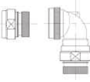
CIR06...straight CIR08...90°
