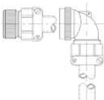
CIR06...straight CIR08...90°
