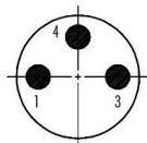
Stifteinsatz M8 Male insert M8
