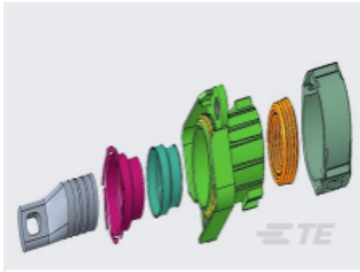
TE Part #YIPT-1PXI-70MM-000 IPT-1pxi 70sqmm
