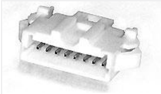
TE Part # 1-292231-3 1.5 MINI CT SGL V SMT W/O BOSS
