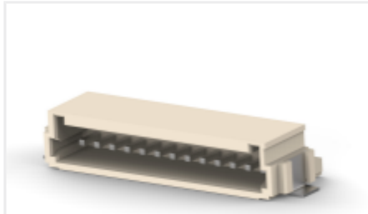
TE Part # 6-292228-3 1.5 MINI CT SGL H SMT W/O BOSS
