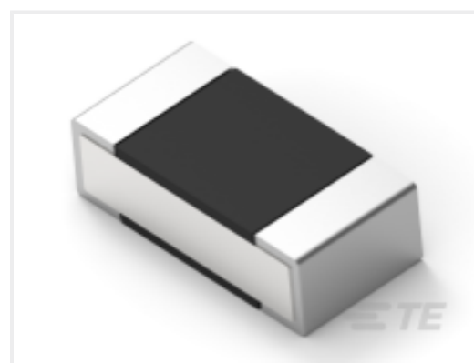
TE Part #5-2176308-0 RP 1E 0.1W 7R5 0.1% 25PPM 1K RL
