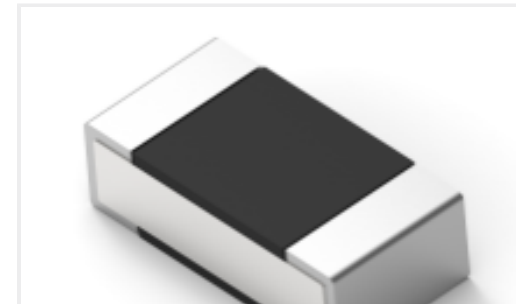
TE Part #2-2176308-2 RP 1E 0.1W 221K 0.1% 25PPM 5K RL
