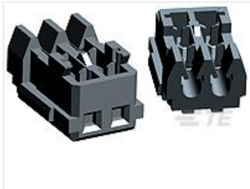
TE Part # 6-353293-3 MINI CT MT REC ASSY 13P BLUR
